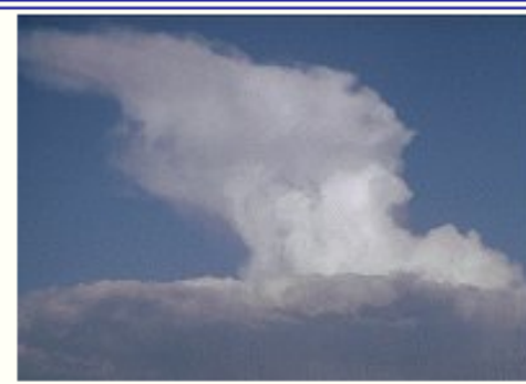
Cumulonimbus
