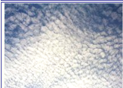
Altocumulus
